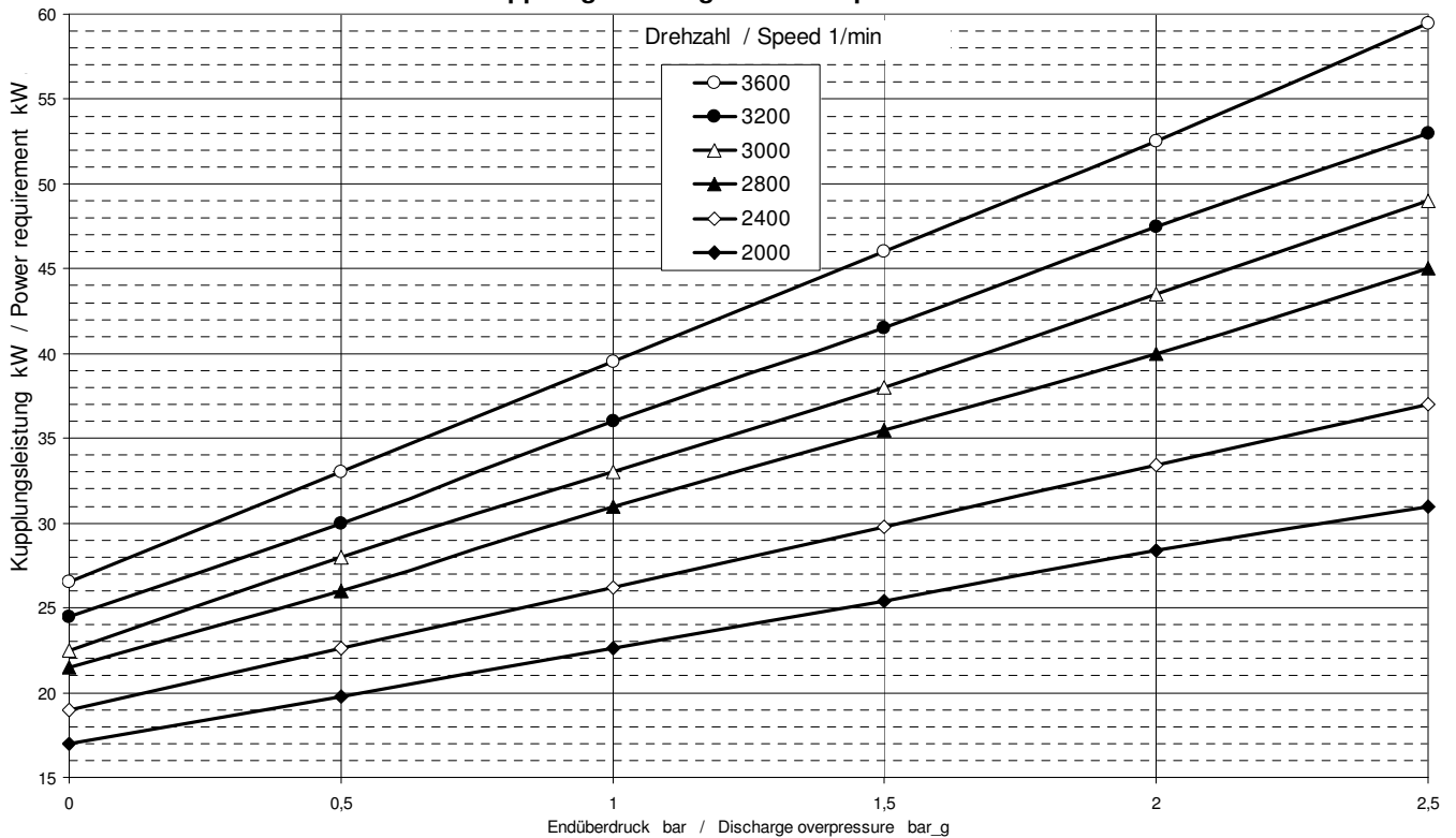
Kupplungsleistung / Power requirement
