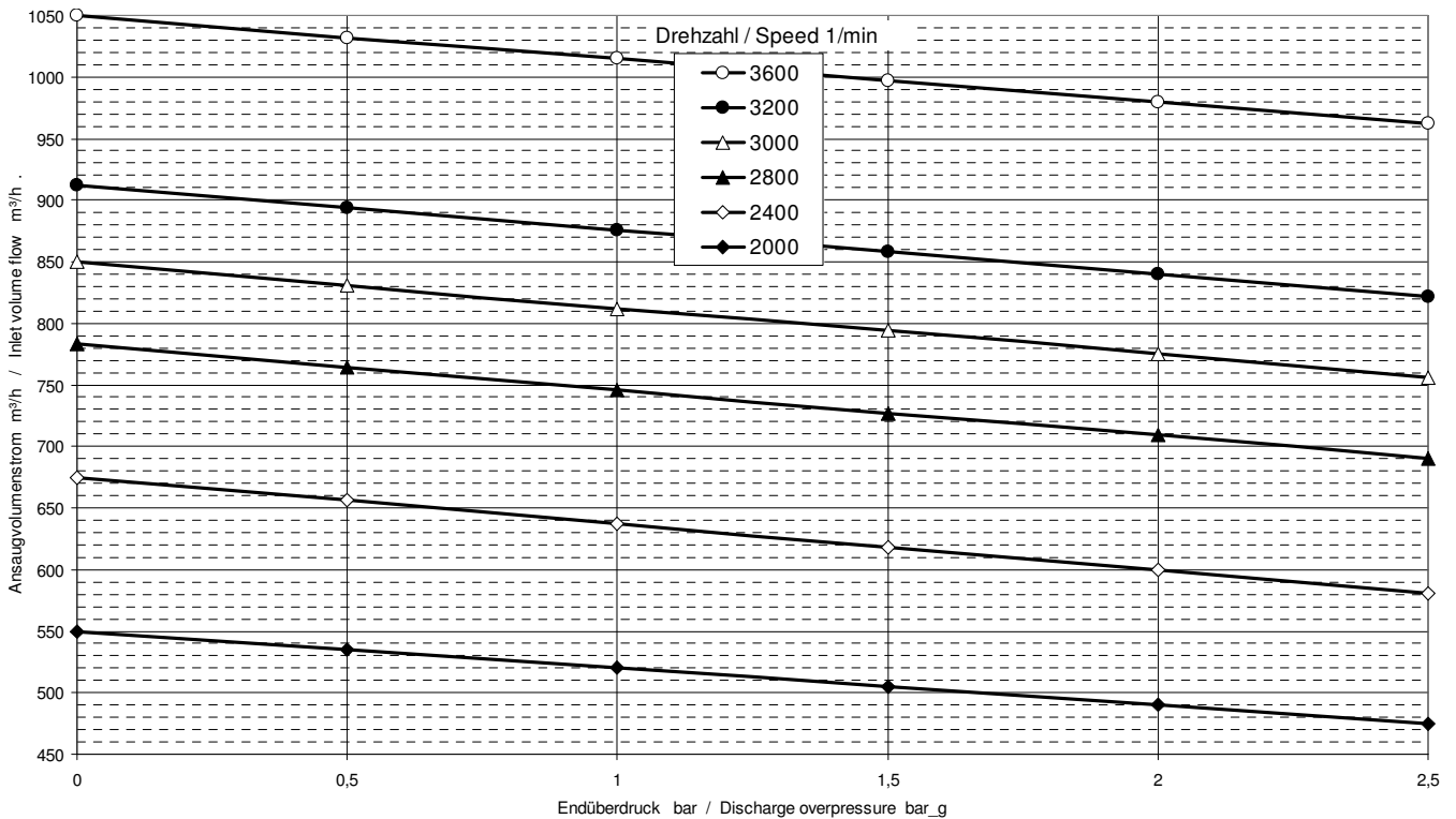
Ansaugvolumenstrom / Inlet volume flow
